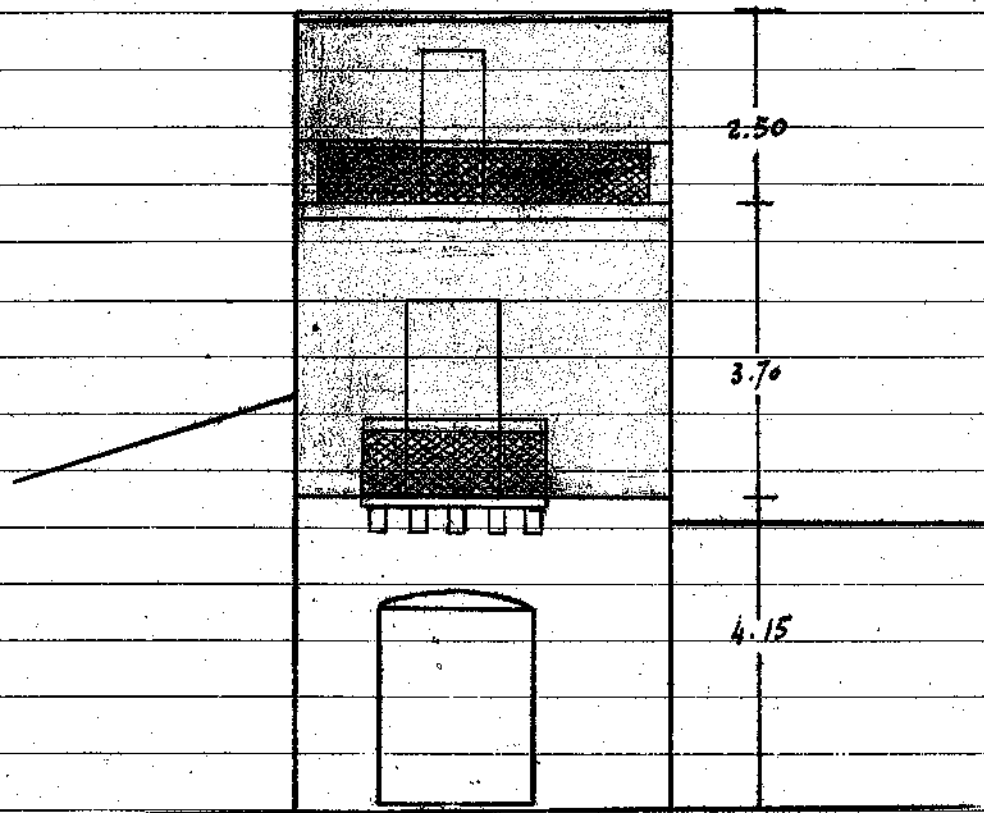
Prospetto
