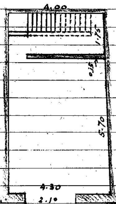
Pianto p.t.
