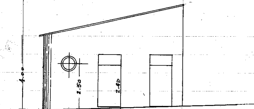
Prospetto Via Circonvallazione
